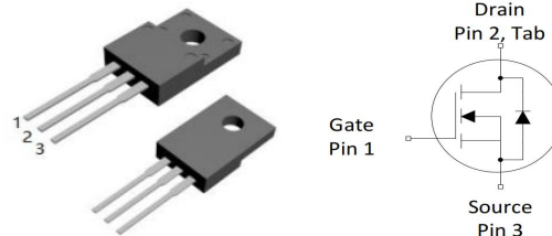
TO-220TF-3L
