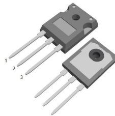
TO-247-3L
