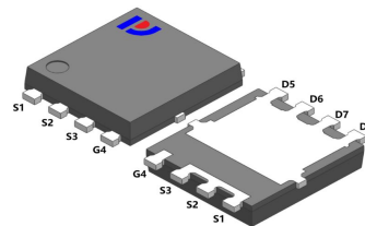
UPDFN5*6-C
