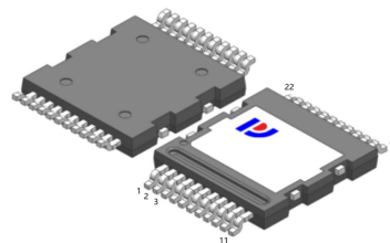
QDPAK
