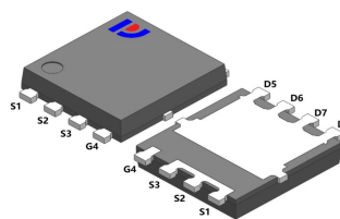
UPDFN5*6-C
